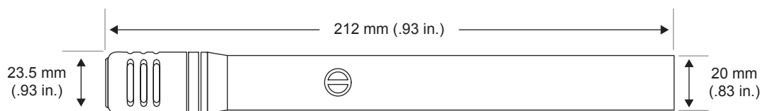
OVERALL DIMENSIONS – DIMENSIONS HORS TOUT GESAMTABMESSUNGEN – DIMENSIONES TOTALES – DIMENSIONI TOTALI – 寸法
