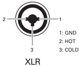
Inputs 1-8
