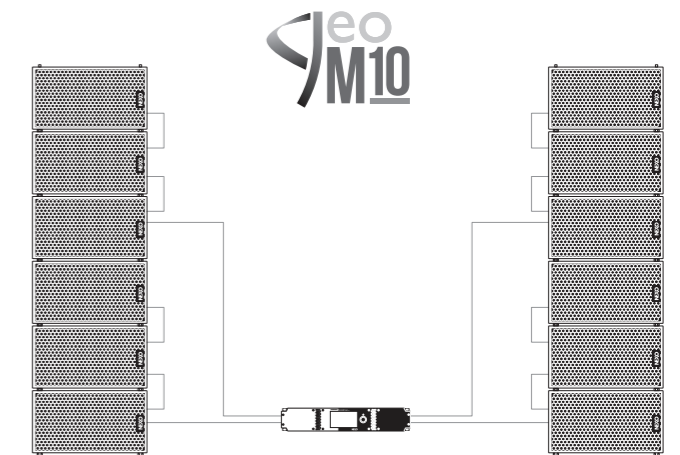
NXAMP4X2MK2 powering 6 X GEO M10 per side
