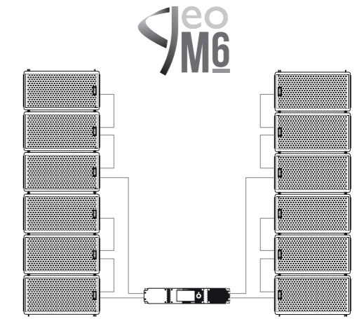
NXAMP4X1MK2 powering 6 X GEO M6 per side
